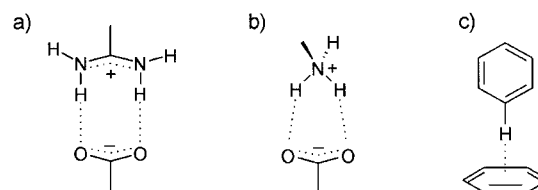
Abbildung 4. Beispiele für spezielle Wasserstoffbrücken: a, b) zweizählige ionische Wasserstoffbrücken (Salzbrücken), c) \text{CH} \cdots \pi -Wechselwirkung.
