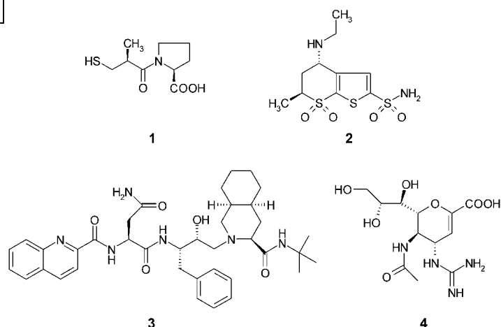
Schema 1. In der Therapie eingesetzte Wirkstoffe, bei deren Entwicklung das rationale Design von entscheidender Bedeutung war.
