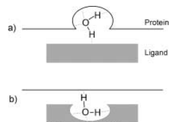
Abbildung 6. Schematische Darstellung von Wassermolekülen, die Protein und Ligand verbrücken; a) häufigerer Fall, bei dem das Wassermolekül stärker an das Protein gebunden ist; b) stärker an den Liganden gebundenes Wassermolekül (Abdruck in veränderter Form nach Lit. [277]).
