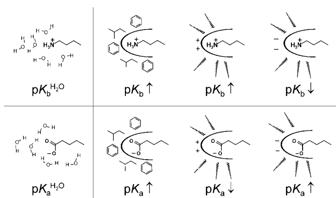
Abbildung 3. Einfluss der Proteinumgebung auf die pK_b -Werte einer basischen (obere Reihe) und die pK_a -Werte einer sauren Ligandengruppe (untere Reihe) im Vergleich zur wässrigen Umgebung ( pK_b^{\text{H}_2\text{O}} , pK_a^{\text{H}_2\text{O}} ).
